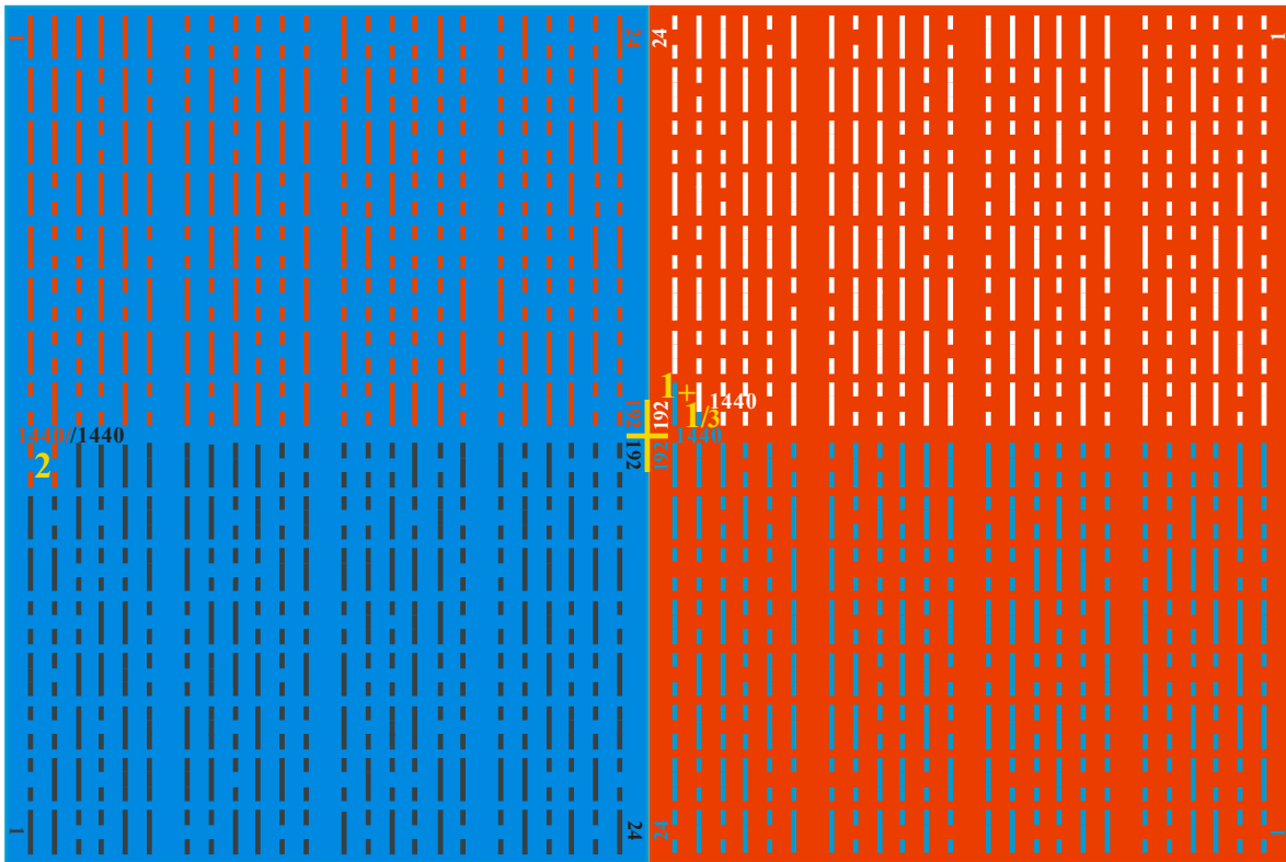
Рис 4. Расчёт параллакса нашего \parallel Мира. Длина сплошной “---” линии = 9 (3+3+3); длина прерванной “- -” = 6 (3+0+3). Сумма длин каждой из четырёх разноцветных групп линий, полученных равновесным делением ( ЗС ) 384 линий гексаграмм И Цзин по обе стороны КСП , равна 1440 . При этом на светлой стороне КСП точка ЗС смещена на 2 линии относительно креста 192/192 \parallel 192 \setminus 192 , а на тёмной стороне на 1 + 1/3 линии.
