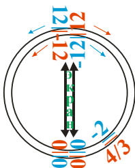
Рис 5. Четыре направления перемещения «я» во Вселенной всевозможных || Миров ( 12||-12 - 0||0 - -12||12 ).
