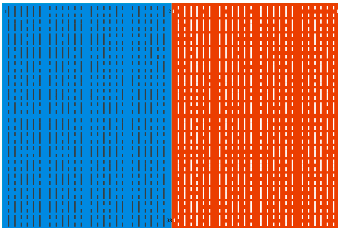
Рис 1. Адресный код нашего мира (одного из 64! || миров) и его зазеркалья. На светлой странице листа КСП знаток И Цзин тотчас же обнаружит классическую последовательность гексаграмм Вэнь-вана.
